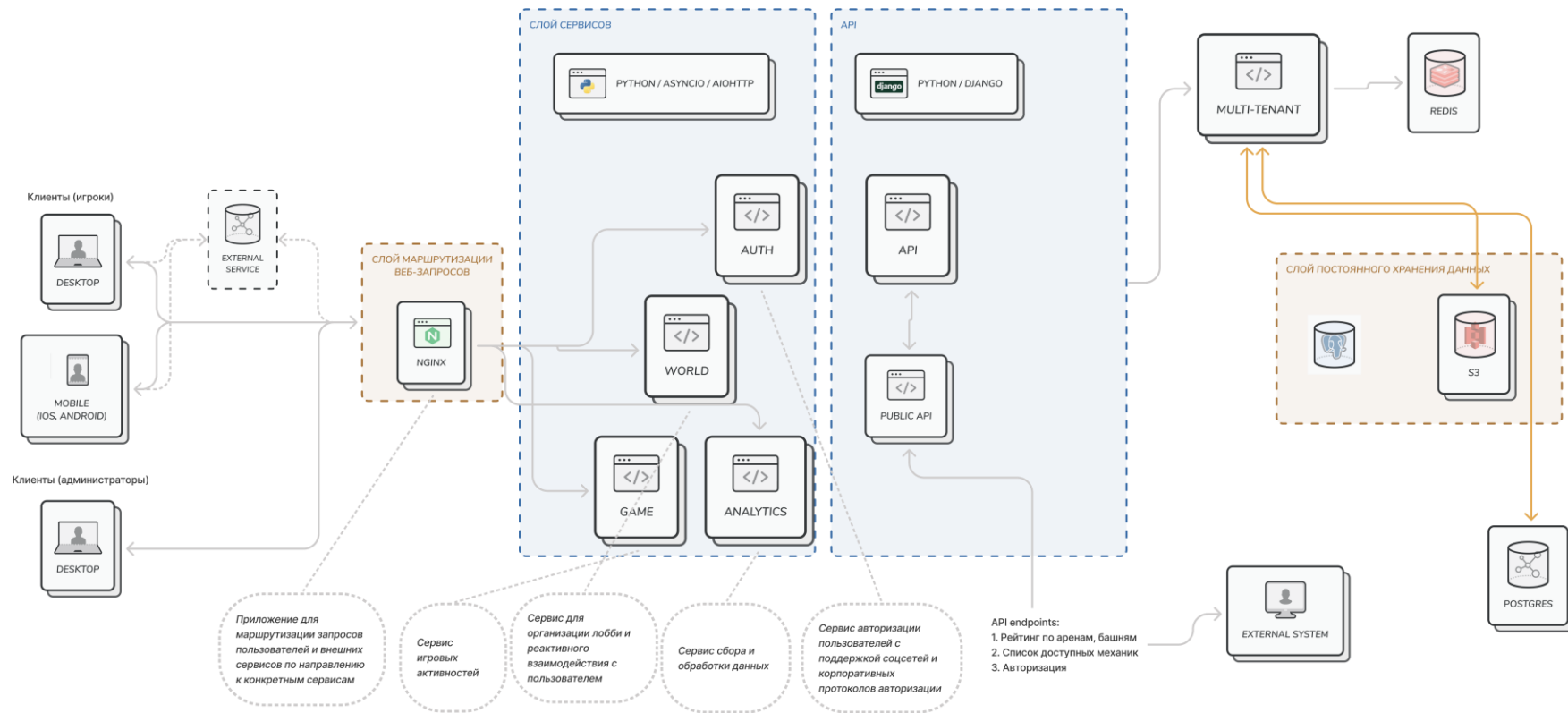
Рисунок 1. Архитектура системы Вовлекай
