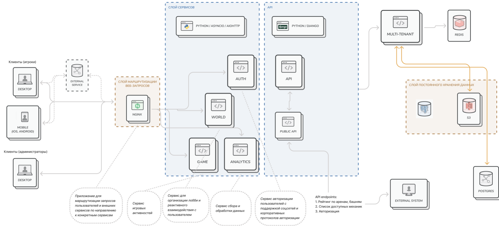
Рисунок 1. Архитектура системы VoxBattle
